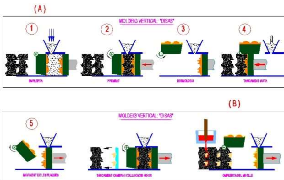
Esquema procés moldeig de sorres i colada
