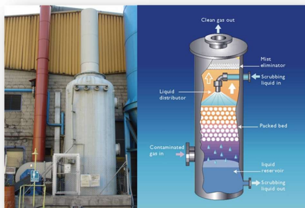
Vista instal·lació scrubber i esquema funcionament
